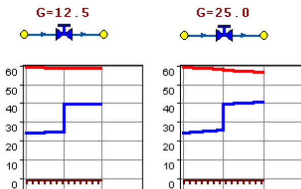
Рисунок 20 – Регулятор давления
