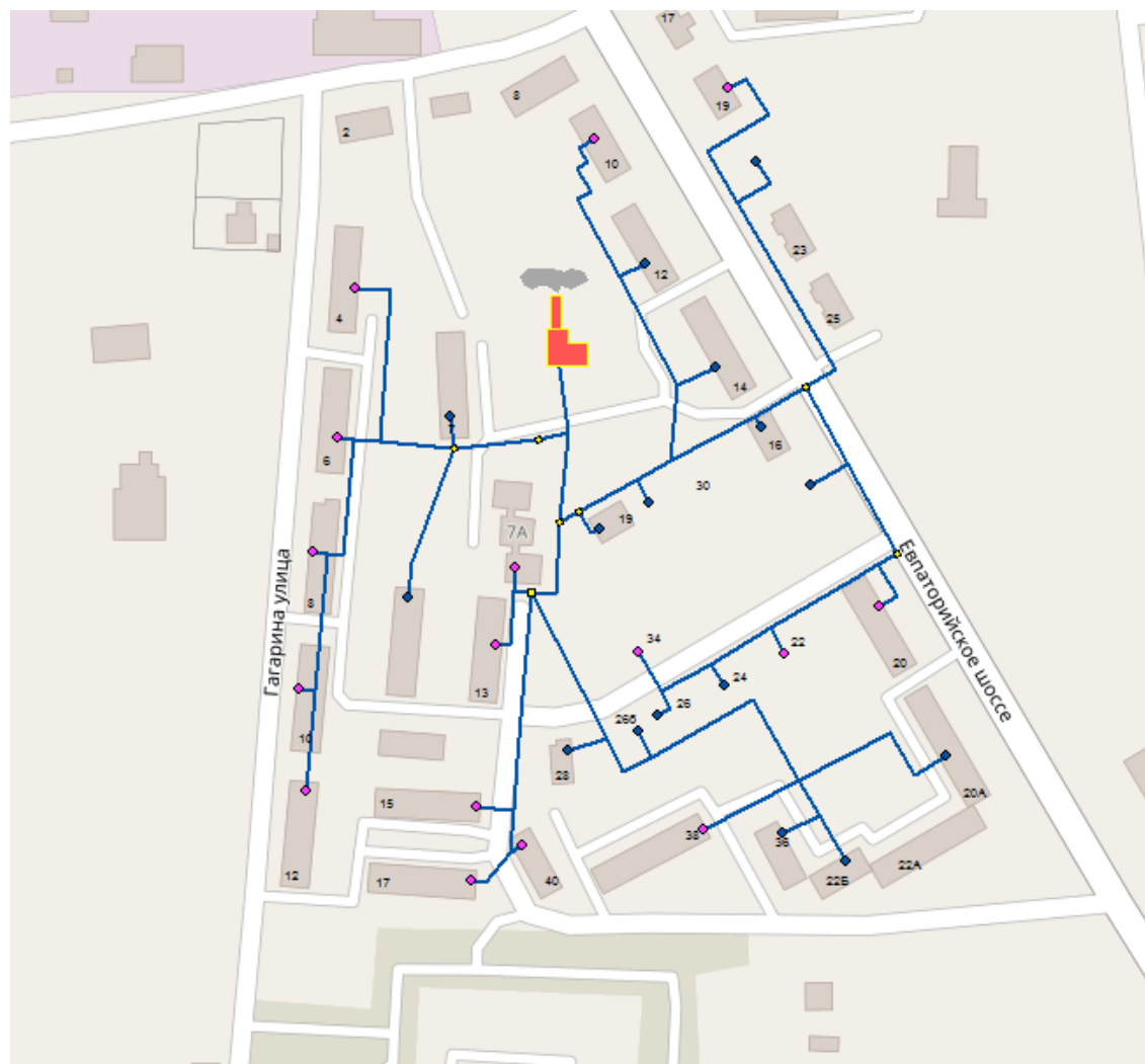
Рисунок 26 – Фрагмент схемы тепловых сетей
