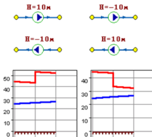
Рисунок 15 – Пьезометрические графики
