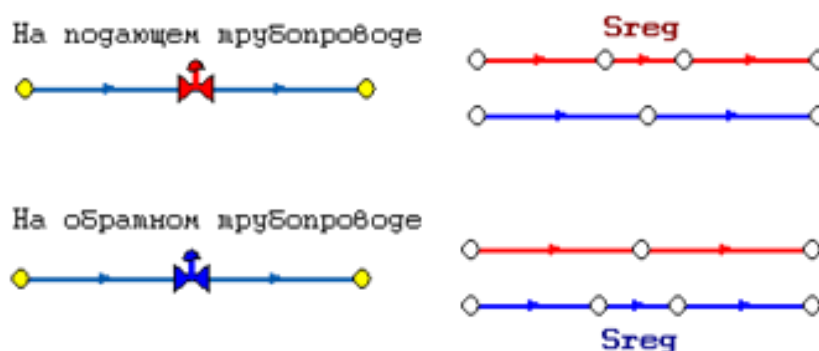
Рисунок 17 – Дросселирующие устройства
